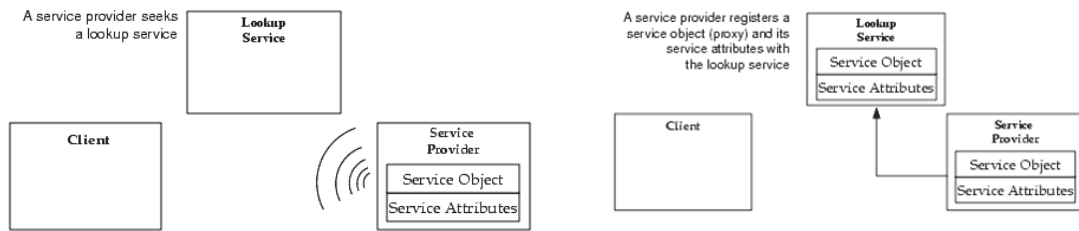
Figura 3.2: Jini - Descoberta e Join (JINI, 2009)
