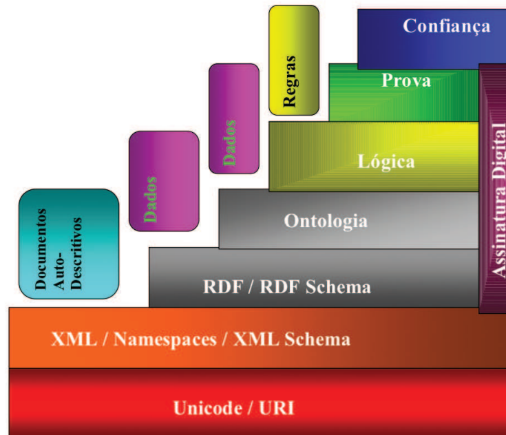
Figura 2.6: Camadas da Web Semântica Proposta pela W3C
