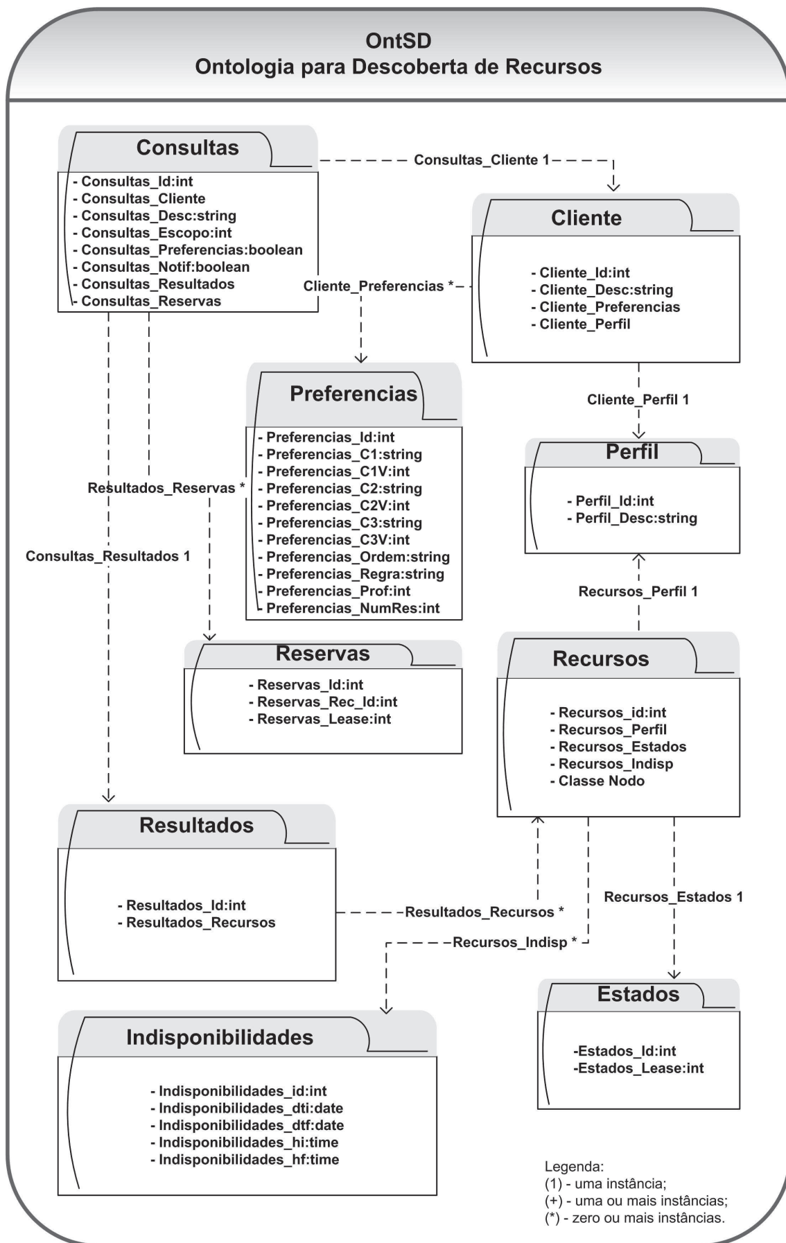
Figura 4.10: EXEHDA-SD: Classes da OntSD
