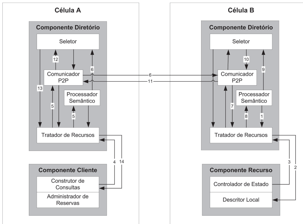
Figura 4.7: EXEHDA-SD: Comunicador P2P
