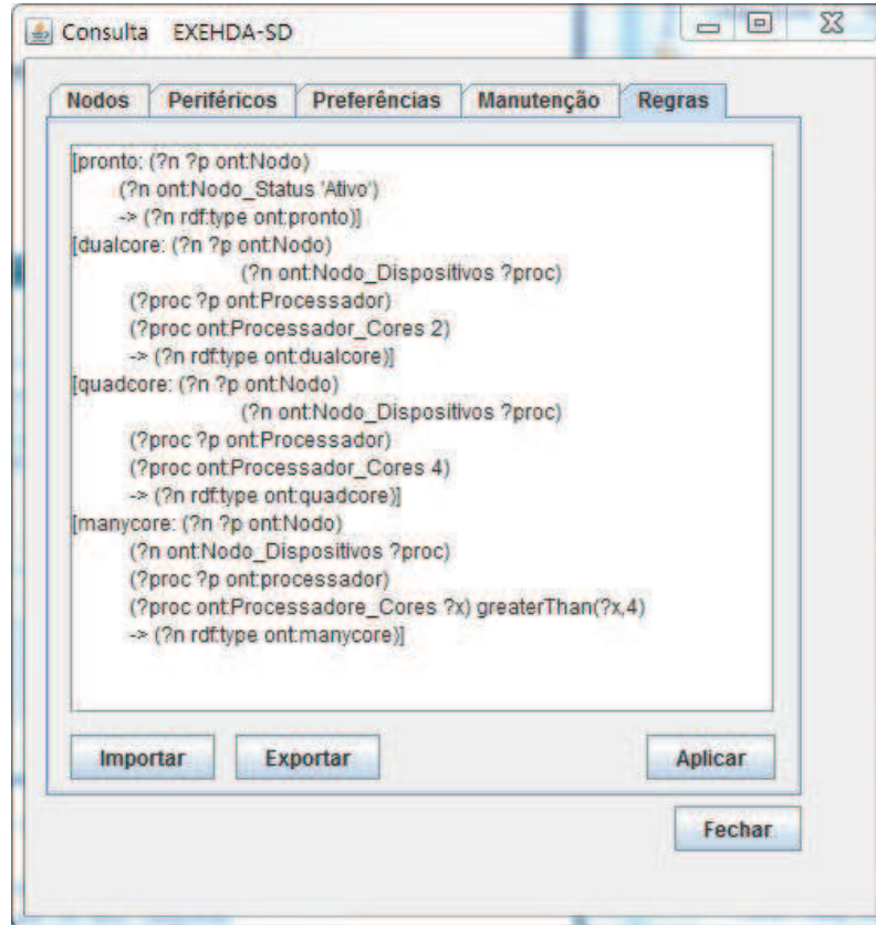
Figura 4.16: EXEHDA-SD: Consulta por Recursos - Regras
