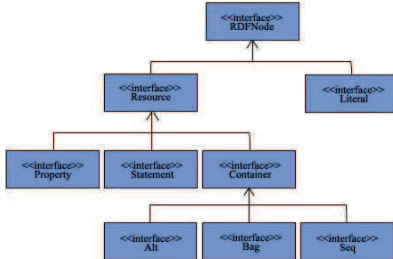
Figura 2.9: Hierarquia de Interfaces da API Jena (VERZULLI, 2001)
