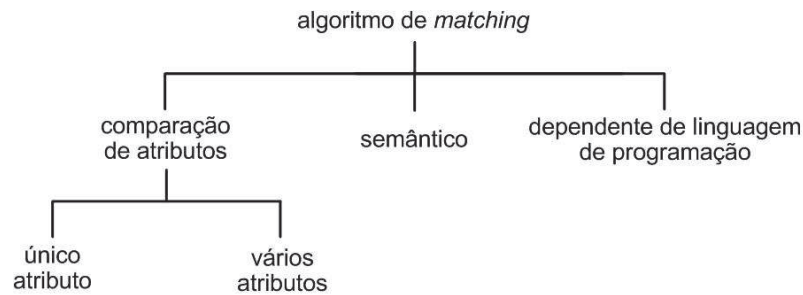
Figura 2.5: Algoritmos de Matching para Consulta por Recursos
