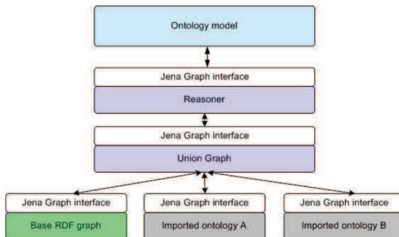
Figura 2.10: Camadas da API Jena (DICKINSON, 2008)
