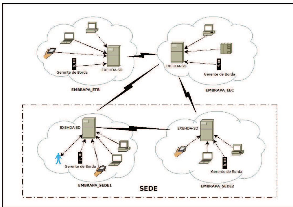
Figura 5.1: CENÁRIO: Organização Celular
