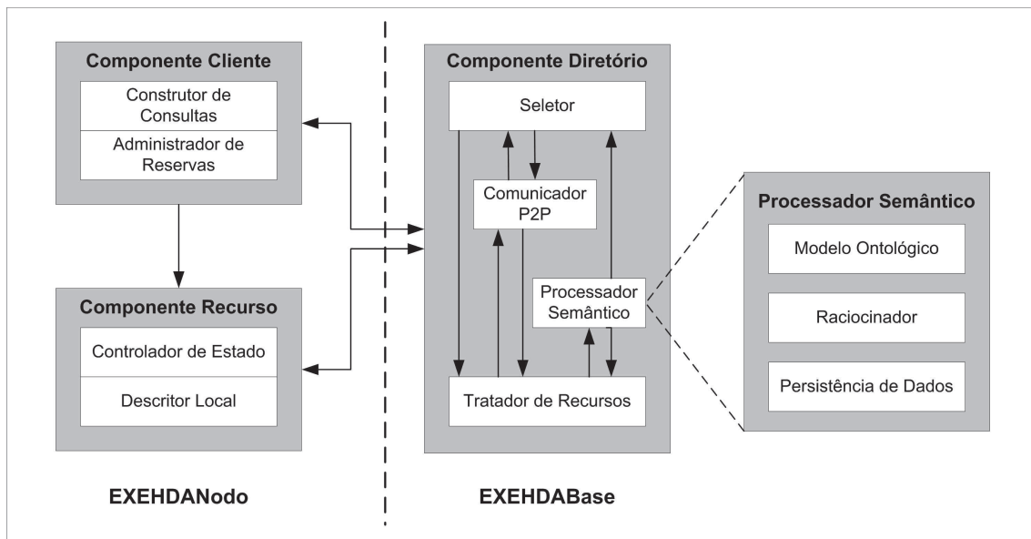
Figura 4.4: EXEHDA-SD: Arquitetura do Modelo Proposto
