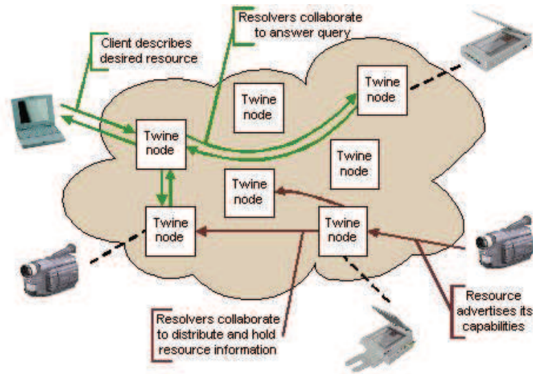
Figura 3.1: Arquitetura INS/Twine (BALAZINSKA; BALAKRISHNAN; KARGER, 2002)
