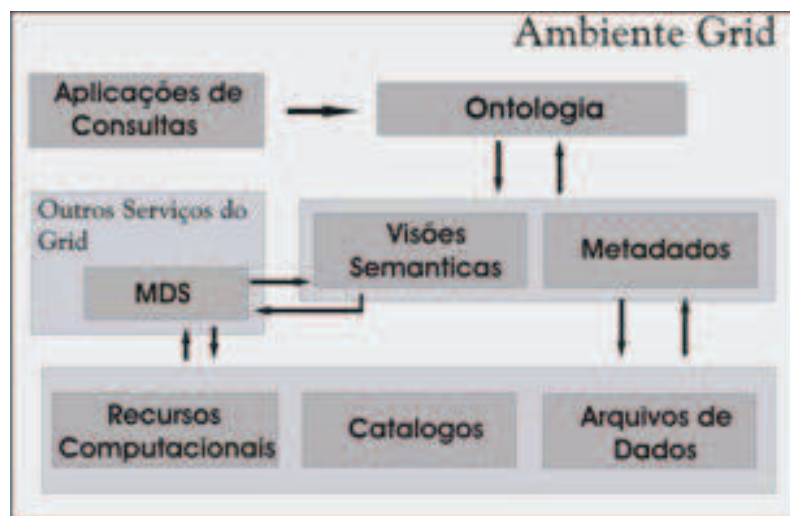
Figura 3.7: Arquitetura de Pernas e Dantas (PERNAS; DANTAS, 2004)
