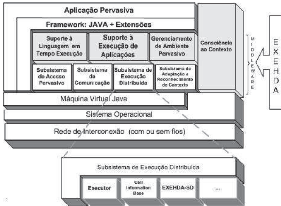
Figura 4.1: Subsistema do EXEHDA Diretamente Relacionado ao EXEHDA-SD
