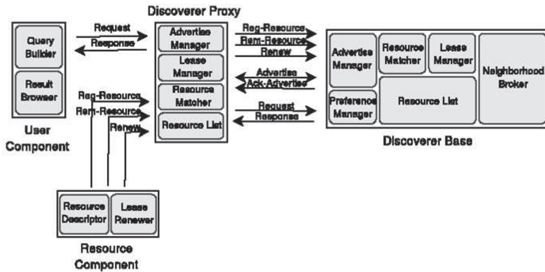
Figura 3.5: Arquitetura PerDis (SCHAEFFER, 2005)
