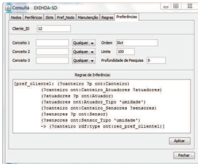
Figura 5.3: CENÁRIO 1: Preferências do Cliente
