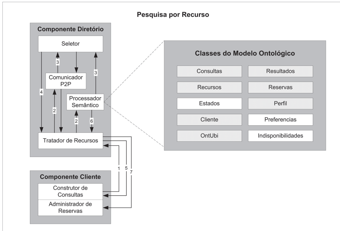
Figura 5.11: CENÁRIO 3: Consulta por Recursos
