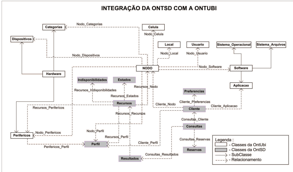
Figura 4.9: EXEHDA-SD: OntSD
