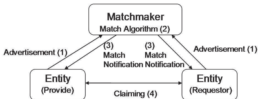
Figura 3.6: Arquitetura Condor (THAIN; TANNENBAUM; LIVNY, 2005)
